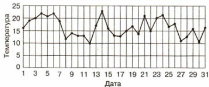
Изменение температуры воздуха в мае 2006 г.
